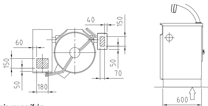
Anslutningar nerifrån
