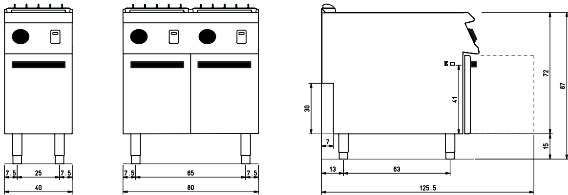
(D) 9222/10 FREM
