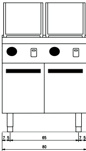
(D) 9423/10 FRGM
