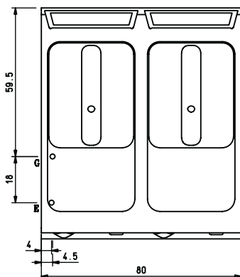
(D) 9423/10 FRGM
