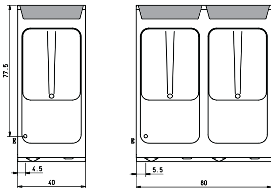
(D) 9222/10 FREM
